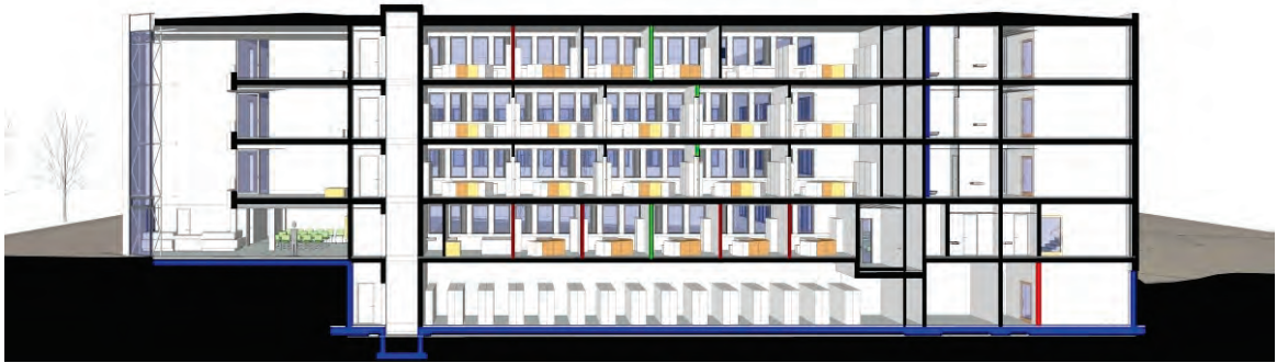
Abbildung 4.27: Aus dem Modell generierter Schnitt (Quelle: schmersahl | biermann | prüßer Architekten + Stadtplaner)
