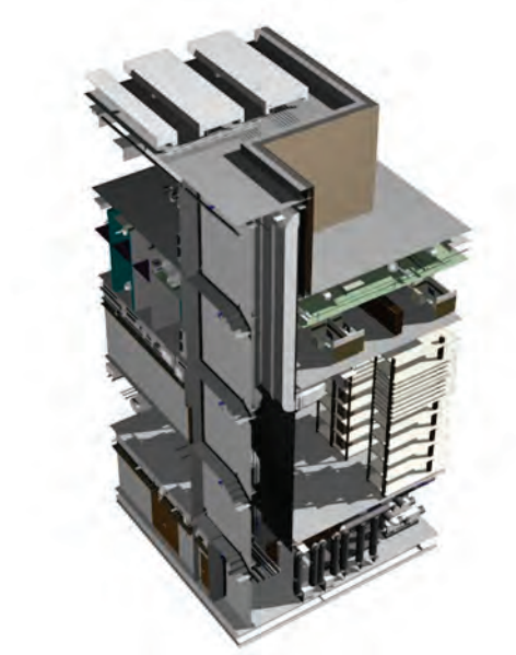
Abbildung 2.2: Querschnitt durch ein Bauwerksmodell Al Ain Hospital (Quelle: OBERMEYER Planen + Beraten)
