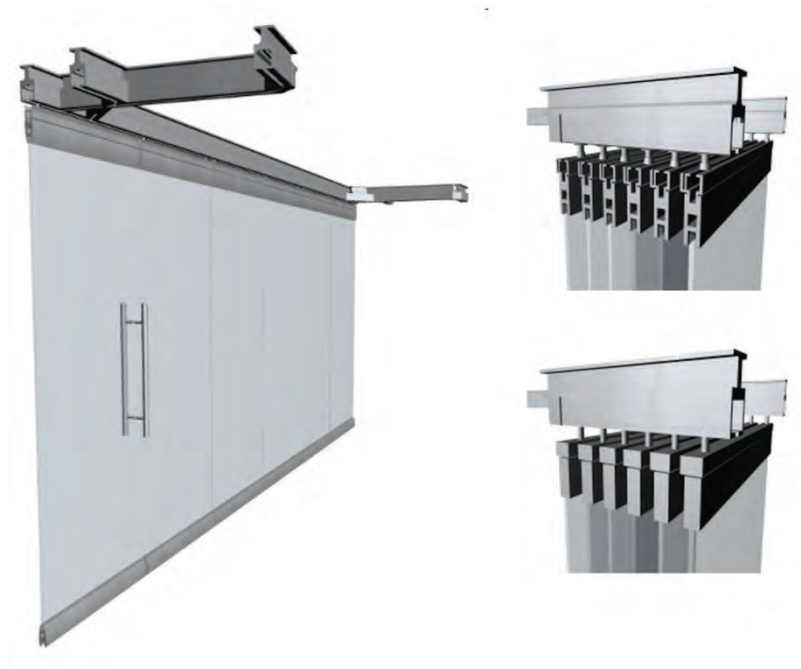
Abbildung 3.7: Beispiel eines vom Bau-Produkthersteller bereitgestellten BIM-Objekts (Quelle: DORMA GmbH + Co. KG)
